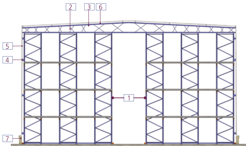
Sección B-B'
